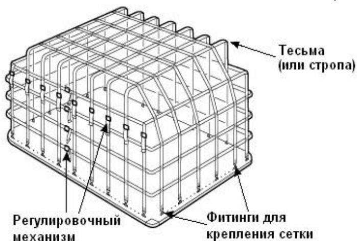
Рис. 3-33 Основные элементы конструкции паллетной сетки, выполненной из строп
