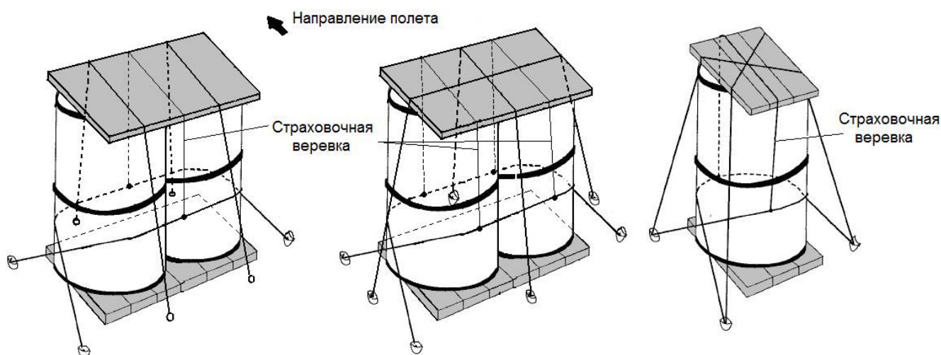
Рис. 3-25 Схемы крепления груза, находящегося в жидком состоянии или сыпучем виде.
