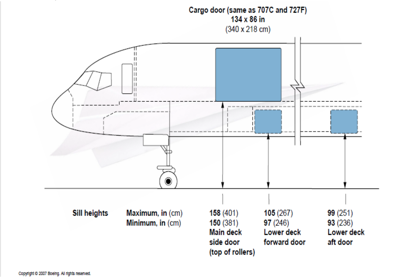
Рис.3-10. Грузовые двери (Cargo doors) Boeing 757 200 PCF
