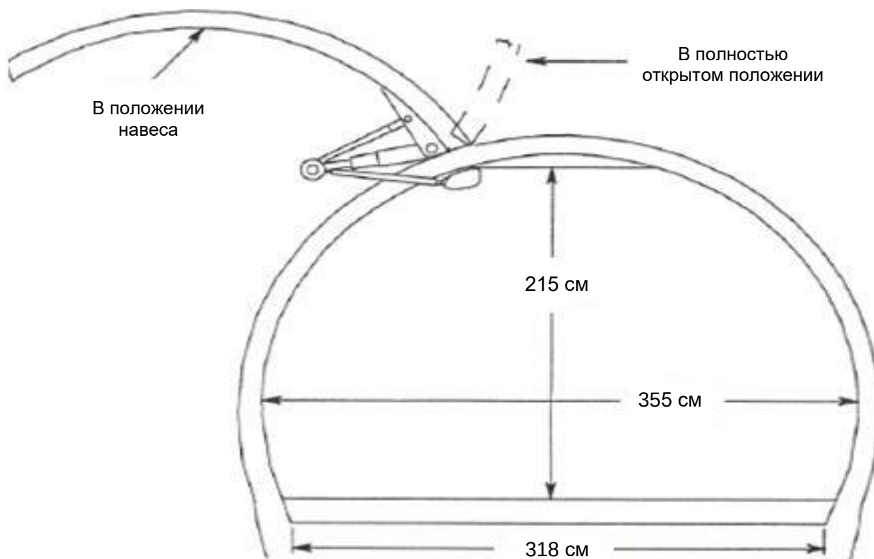
Рис. 3-12. Контуры Boeing 757 200 PCF
