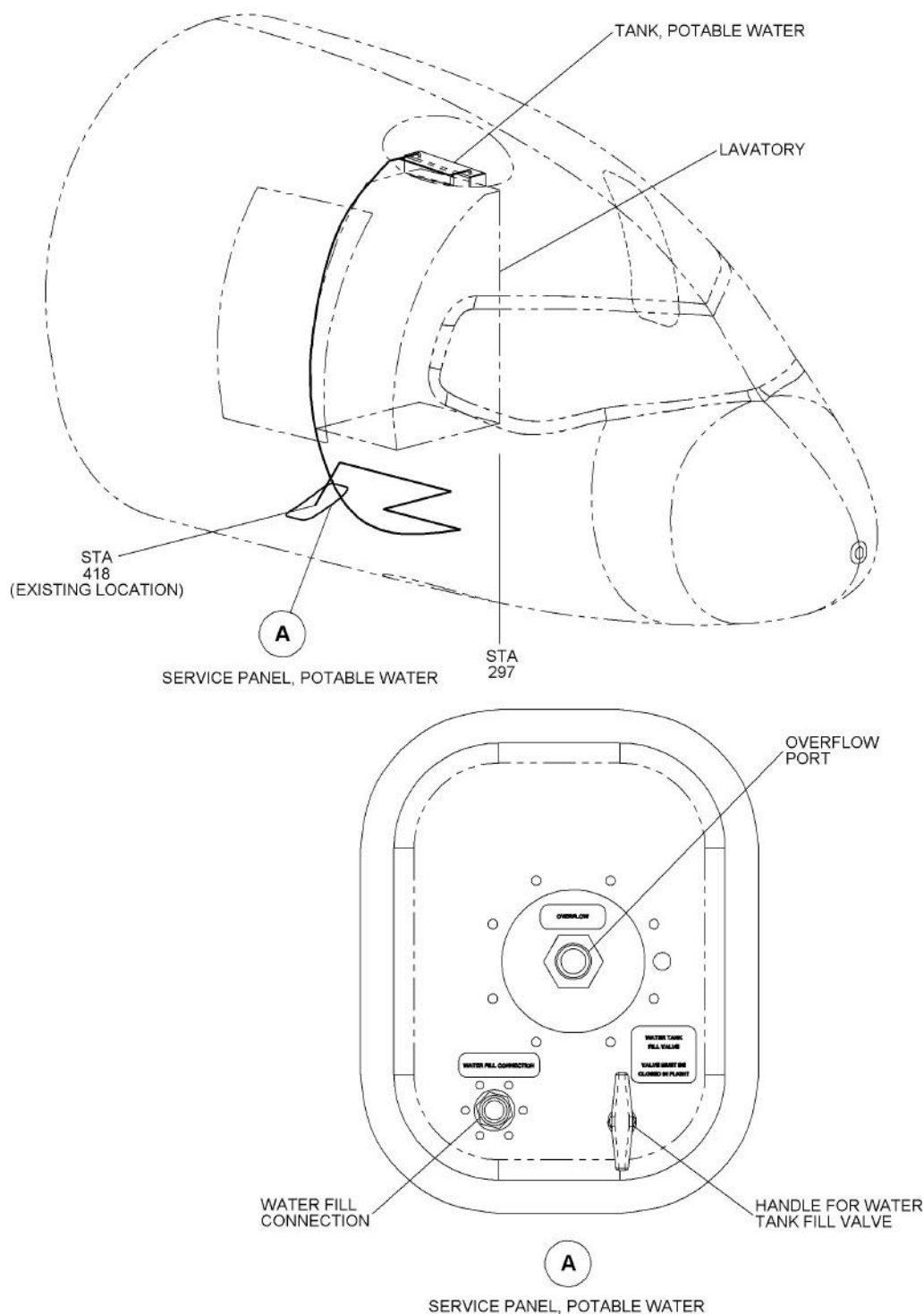
Рисунок 28. Расположение сливной и заправочной панели.
