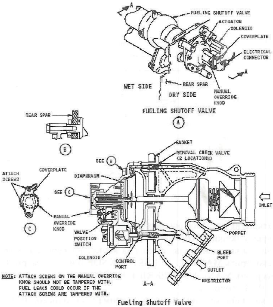
Рисунок 35. Заправочный клапан.
