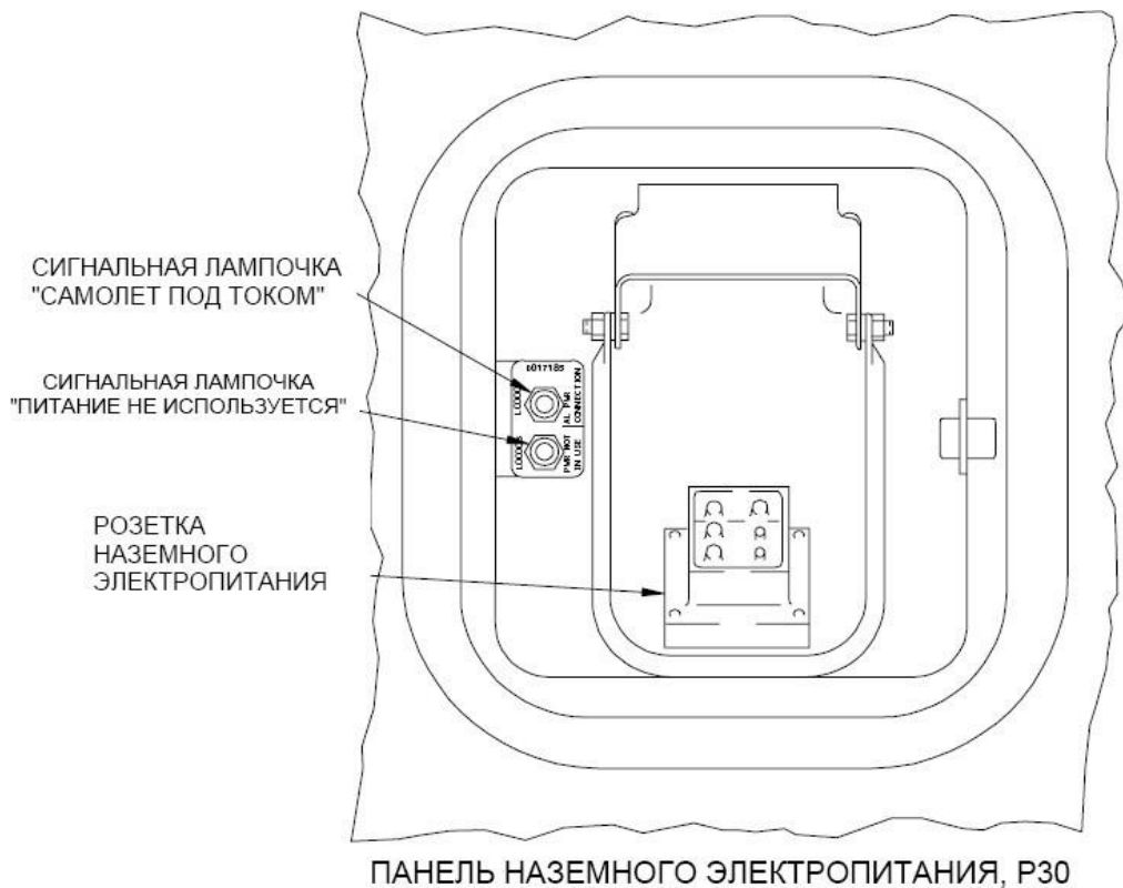
Рисунок 45а. Панель наземного электропитания.
