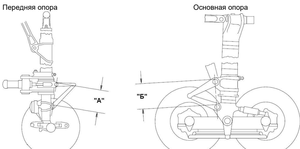
Рисунок 22. Передняя и основная опоры, измерение выхода штоков амортизаторов шасси.
