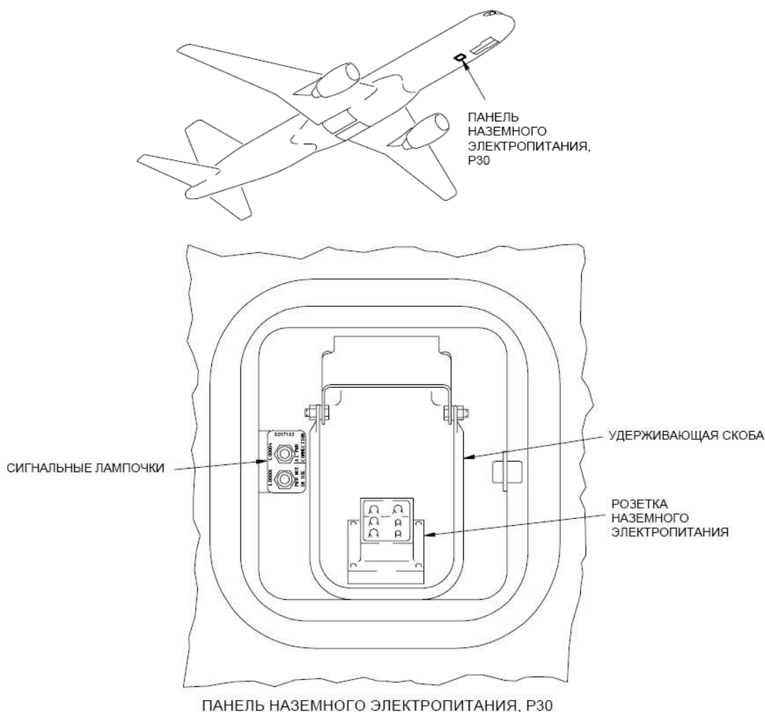
Рисунок 45. Панель наземного электропитания.
