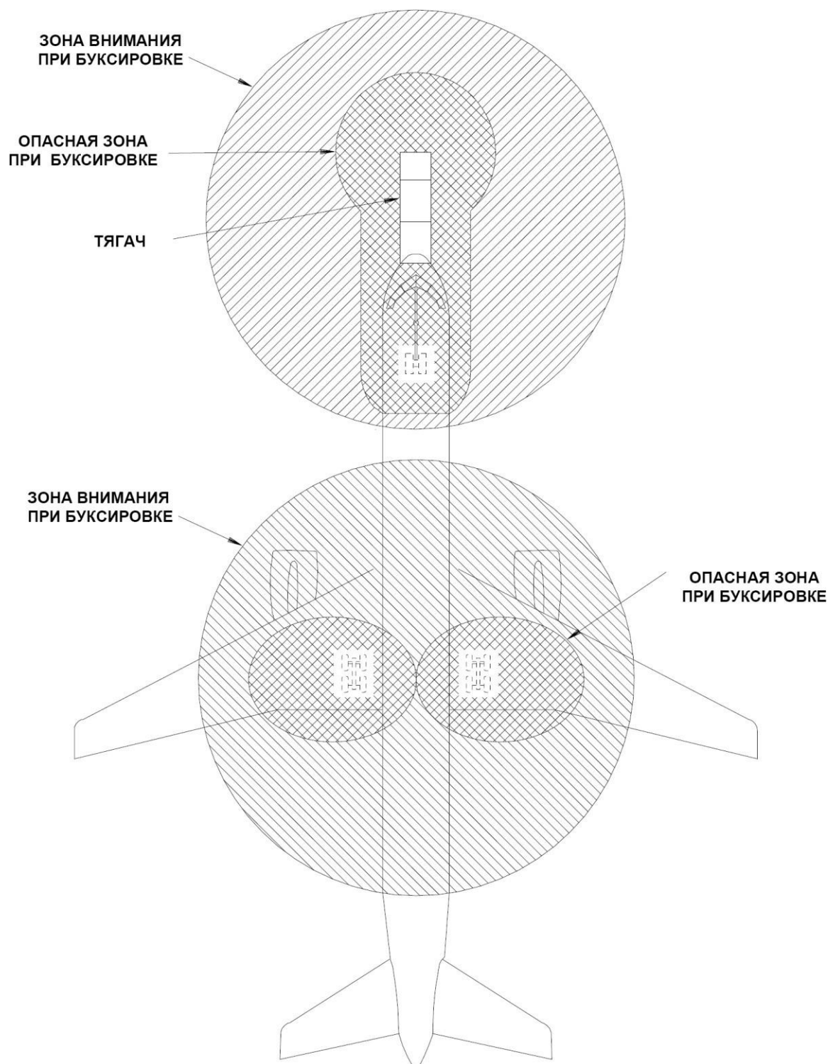
Рисунок 24. Опасные зоны при буксировке
