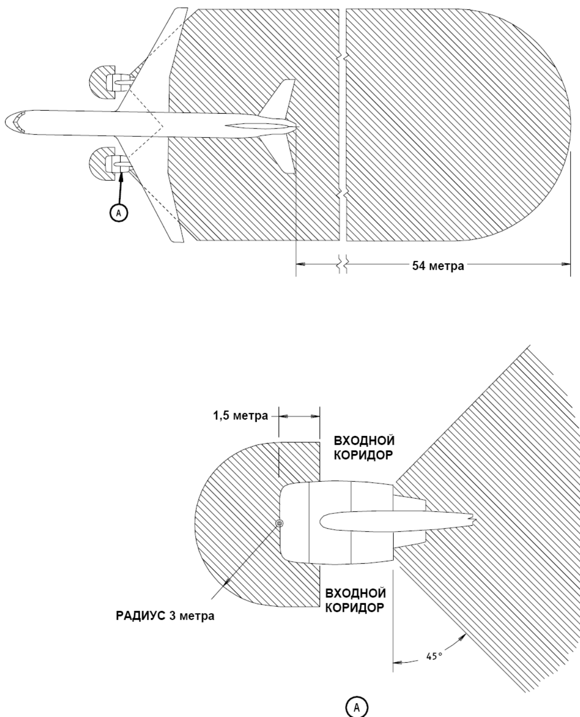
Рисунок 25. Опасные зоны при работе двигателей на режиме малого газа.
