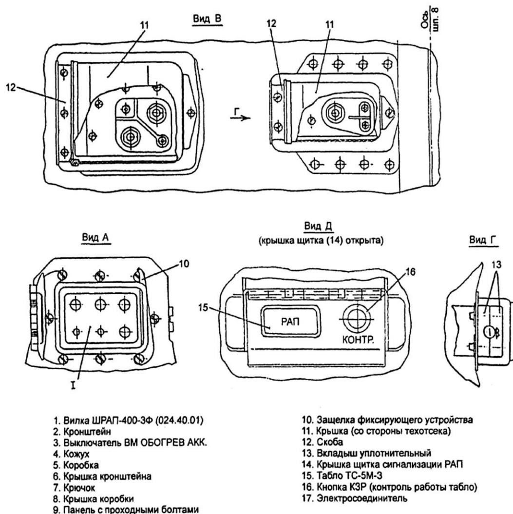
Рисунок 10б. Щиток аэродромного питания и гнездо заземления ВС на стоянке (Ту-204С)
