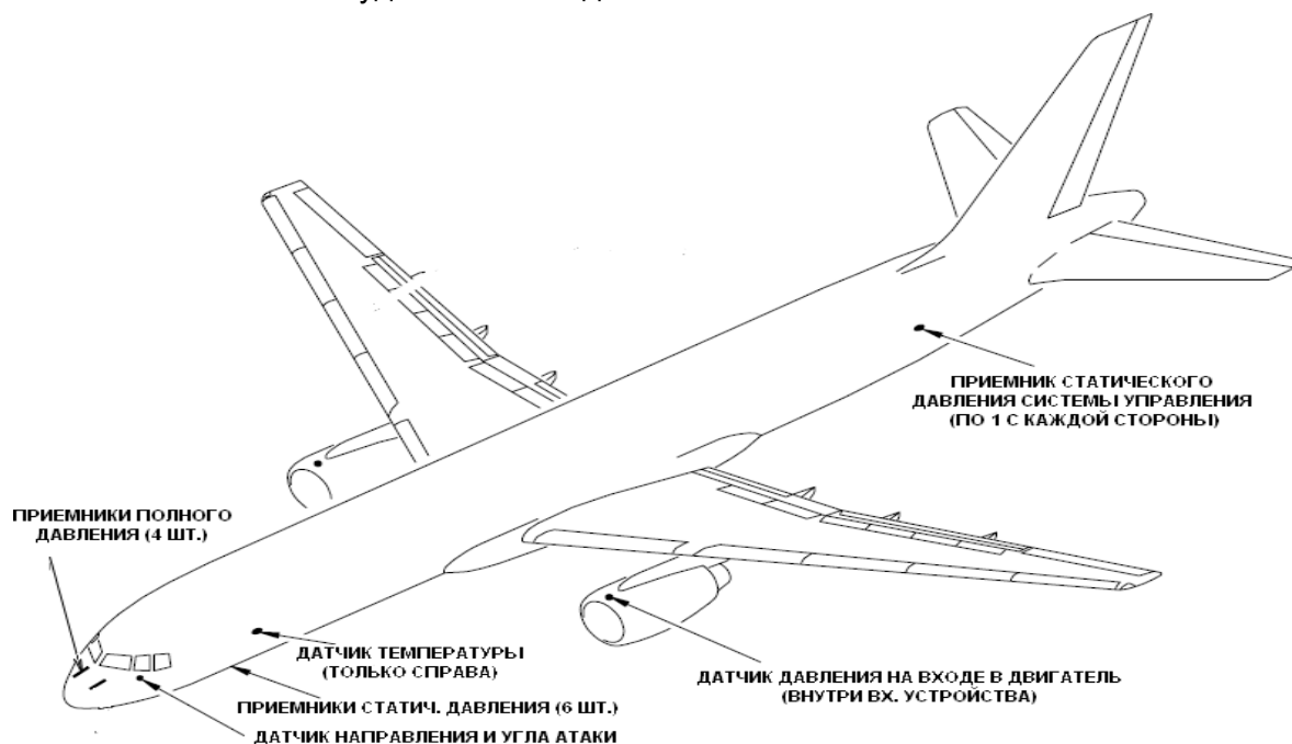
Рисунок 64. Расположение приемников воздушного давления и датчиков.
