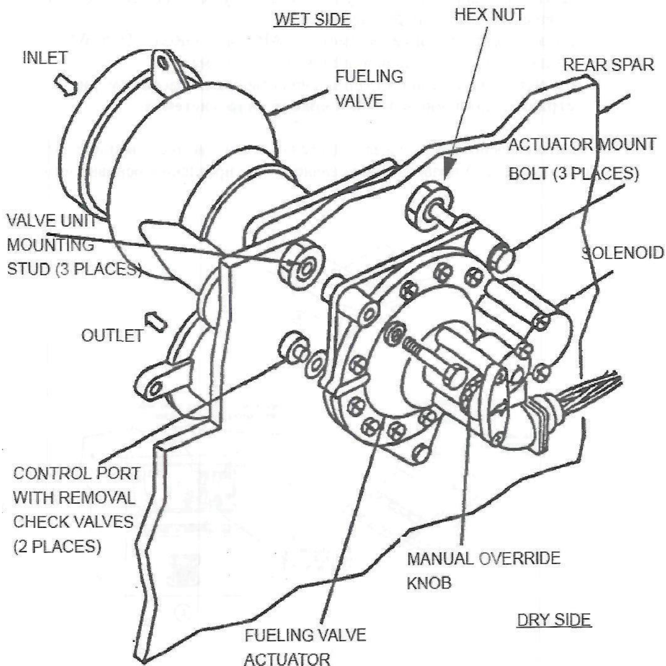
Рисунок 36. MANUAL OVERRIDE KNOB (Кнопка ручной блокировки).
