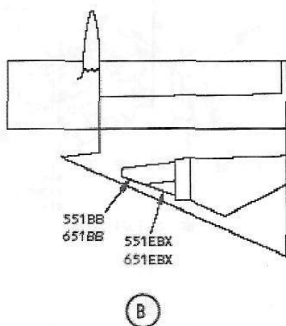
Рисунок 34. Доступ к заправочным клапанам.
