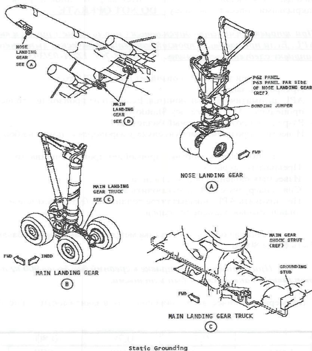
Рисунок 30. Точки заземления на ВС.
