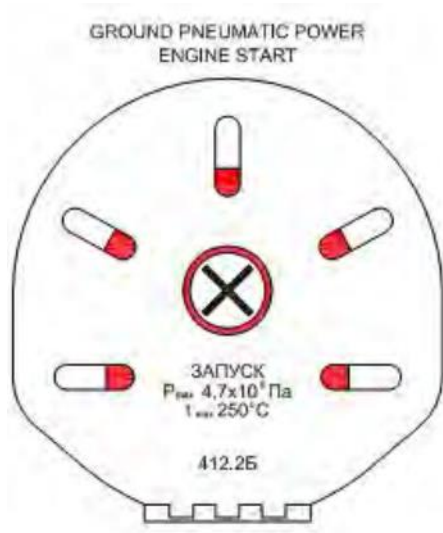
Рисунок 16. Лючок подсоединения штуцера УВЗ наземное обслуживание в неблагоприятных
