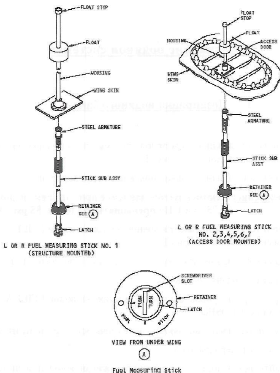
Рисунок 43. Мерные линейки.
