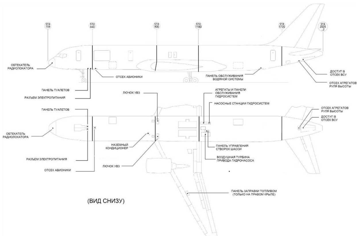
Рисунок 29. Расположение точек сервисного обслуживания ВС
