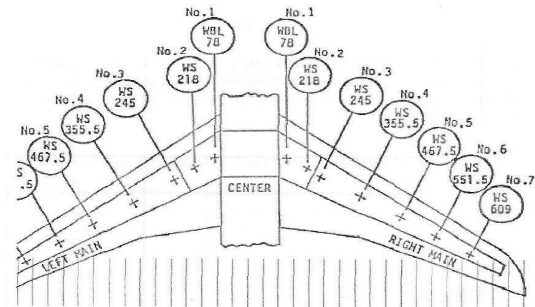
Рисунок 39. Расположение мерных линеек.
