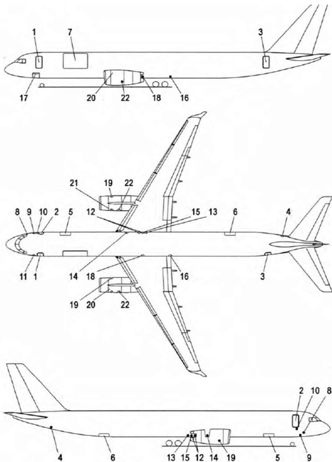
Рисунок 06. Расположение точек ВС используемых при НО.
