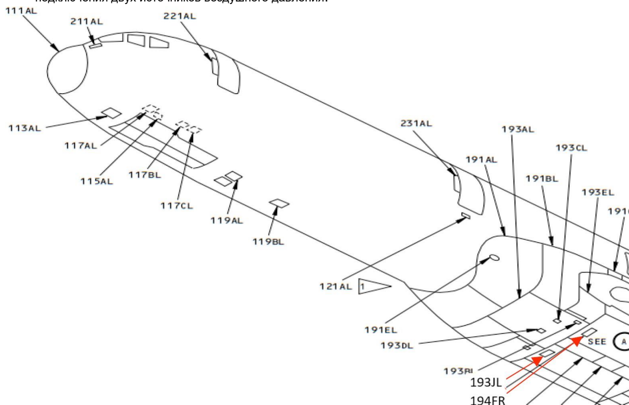
Рисунок 50. Панель доступа к фланцам подключения УВЗ.
