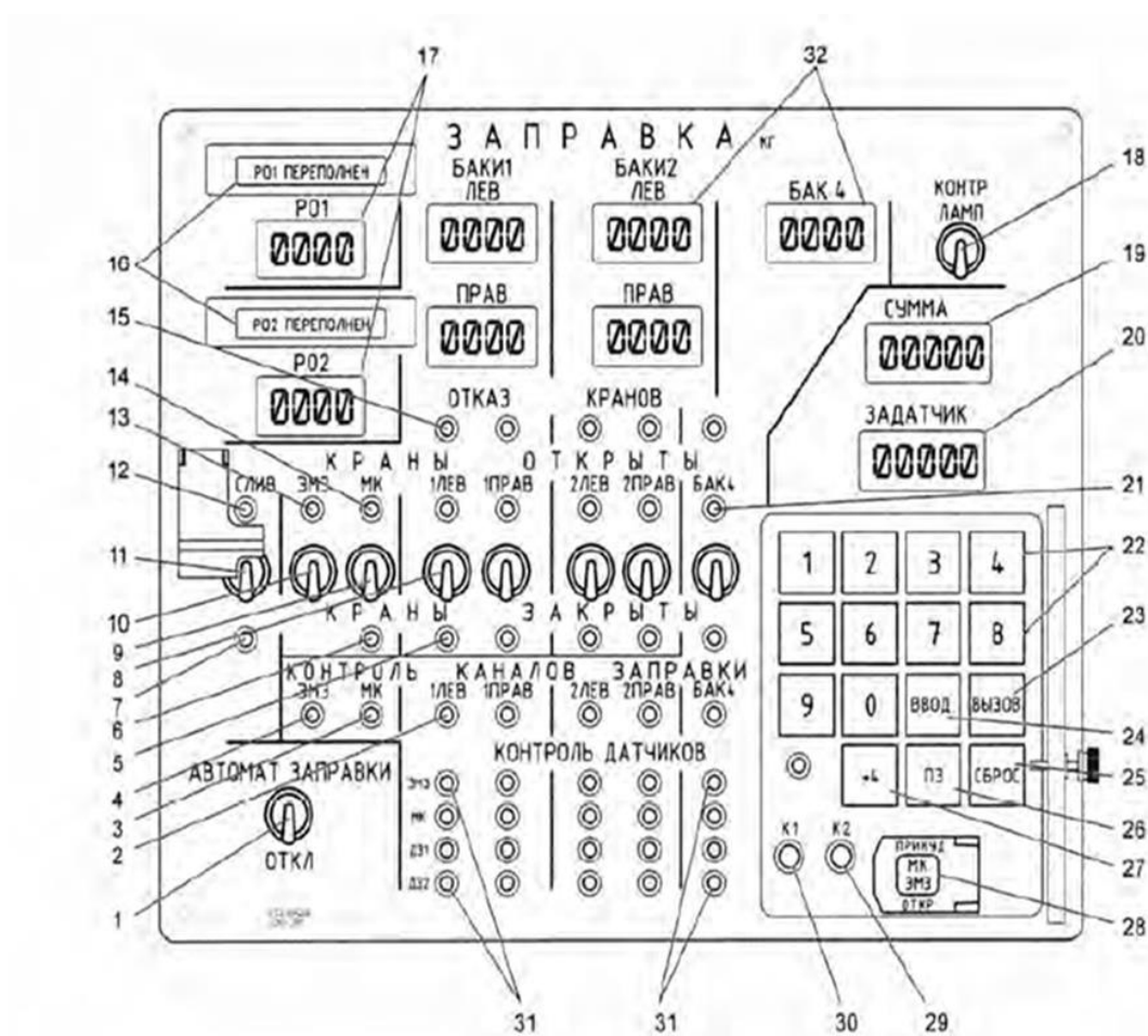
Рисунок 14. Пульт управления заправкой топлива
