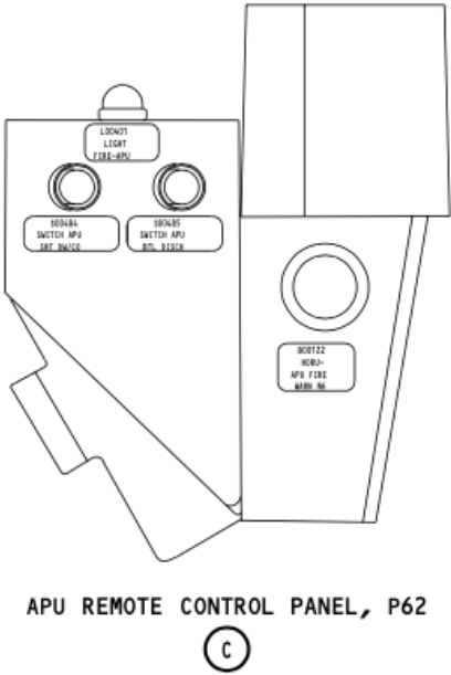
Рисунок 63. APU REMOTE CONTROL PANEL (P62 панель).
